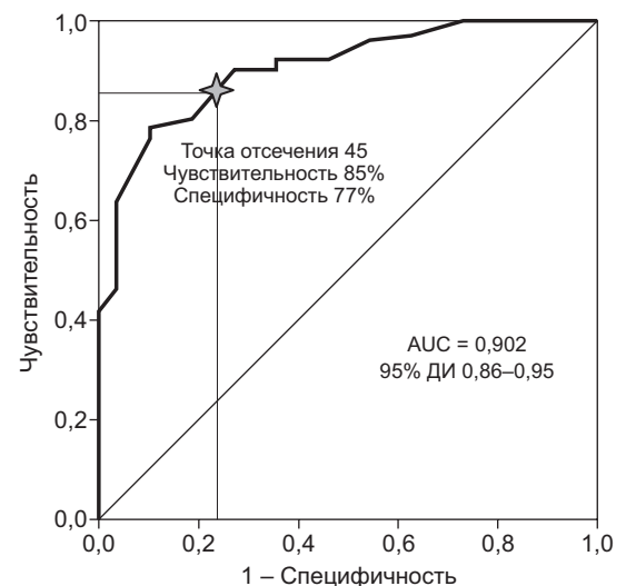
Рис. 2. ROC-кривая алгоритма прогноза вероятности ИКД-терапии.
